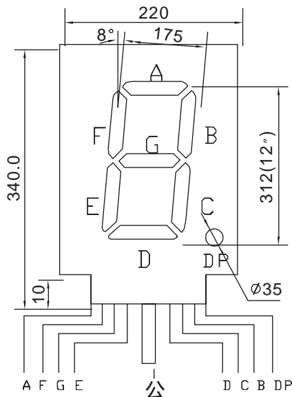
组装板走线图 (反面)
